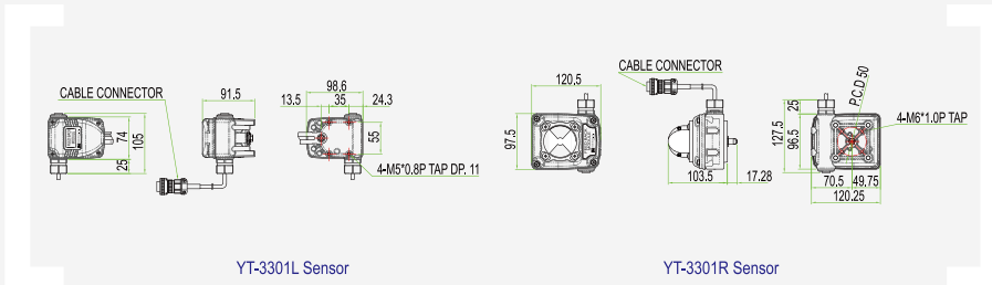
YT-3301 Body
